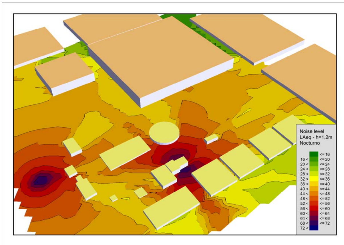
Figura 11: Modelo acústico
