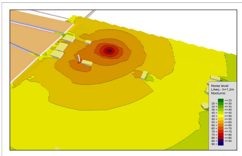
Figura 19: Modelo acústico
